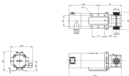
23407 MOBIMAx 54 l/min-14.3 gpm - 24 V-DC-Abgreifklemmen
